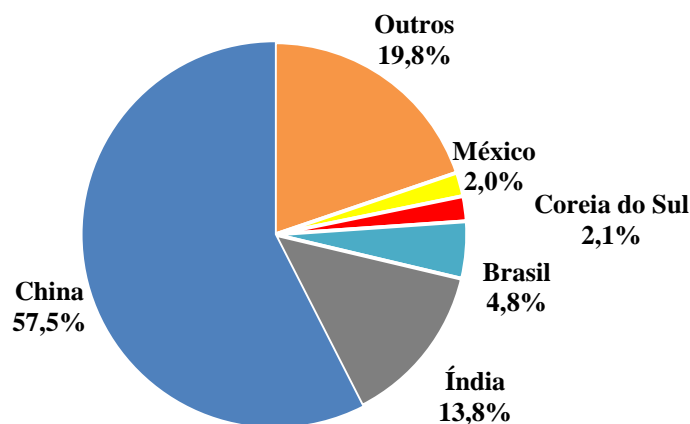
Figura 3 – Estimativa de redução de emissões por países para o primeiro período de obtenção de créditos das atividades de projeto registradas até 30 de setembro de 2014.
