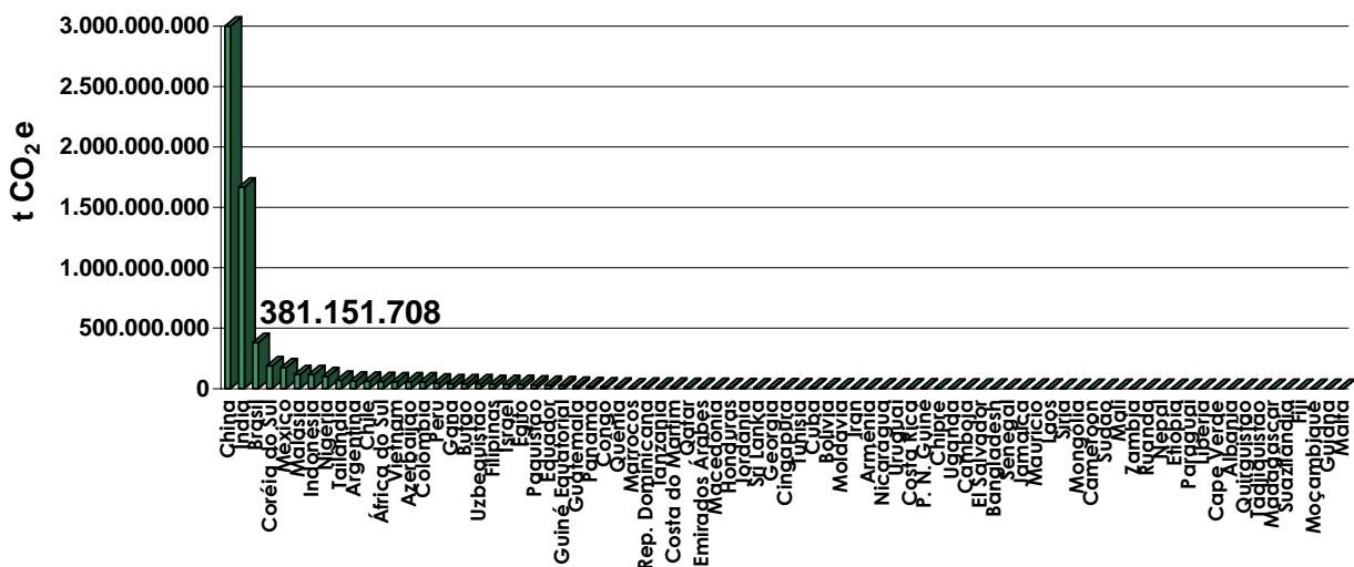
Figura 2 – Potencial de Redução de emissões para o primeiro período de obtenção de créditos
